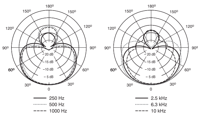
Padrão Polar
